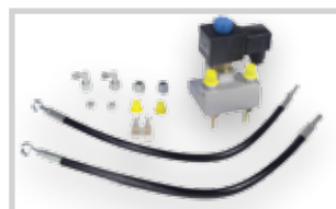
Antipanicové zařízení* umožňuje pohyb ráhna v případě výpadku elektrické energie
